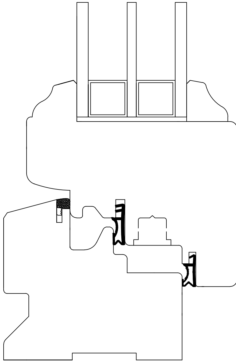
Legno 90 mm ultra - profilo centro storico -
