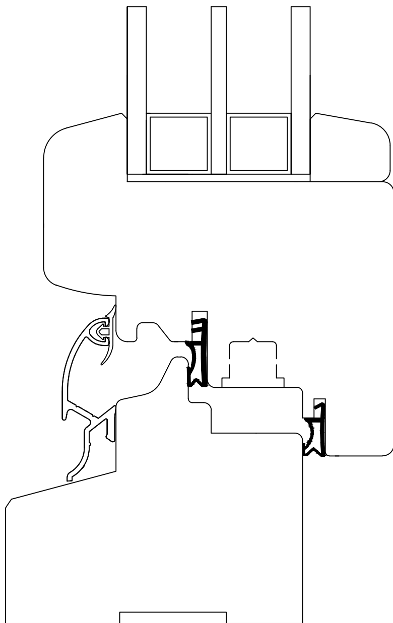
Legno 90 mm ultra - profilo standard -
